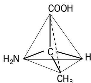
L-アラニン
