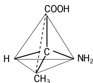
D-アラニン
